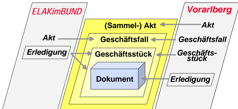
Abbildung 10: Ebenen von EDIAKT II mit zwei Abbildungsbeispielen
