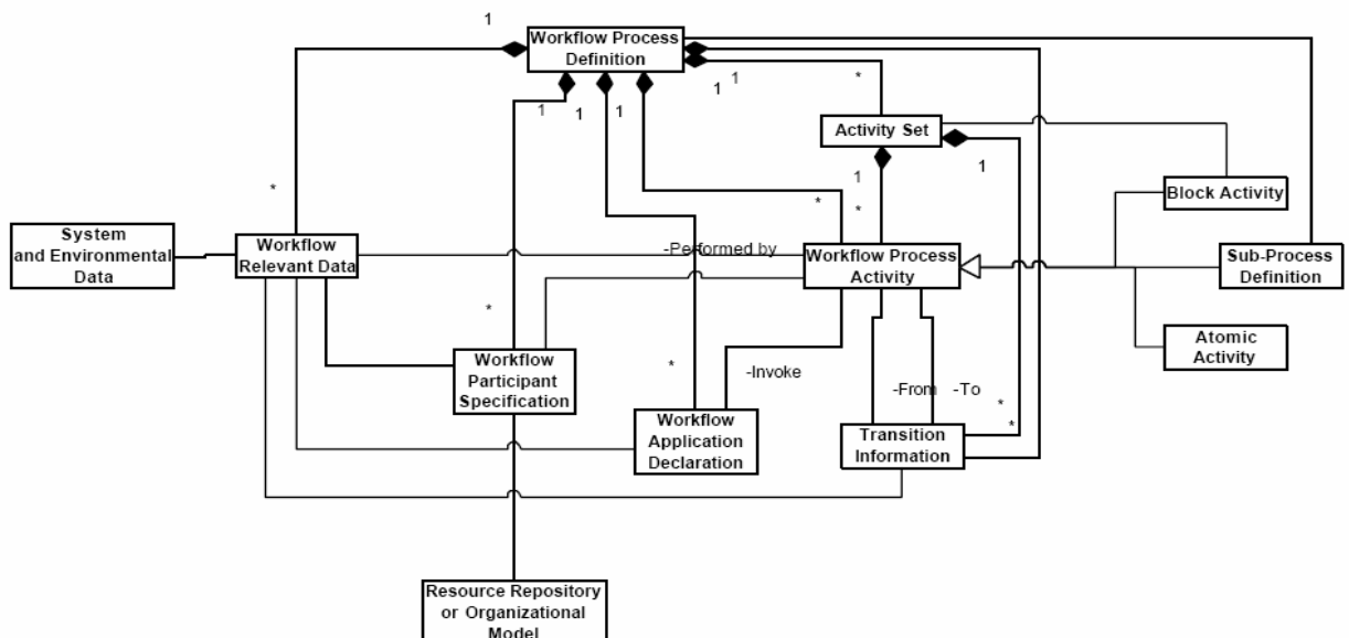
Abbildung 41: Metamodell von XPDL
