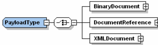
Abbildung 31: Element Payload des Dokuments
